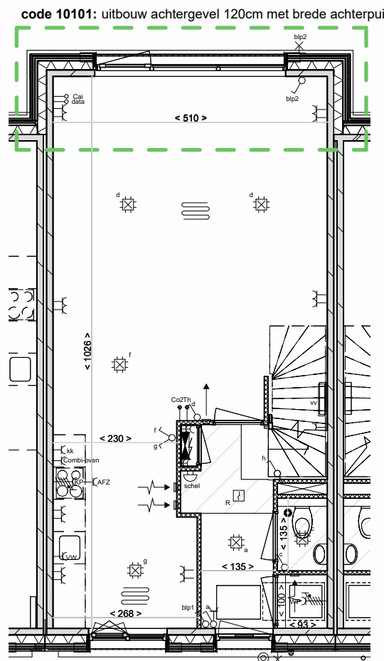
begane grond
