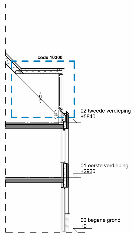
doorsnede
