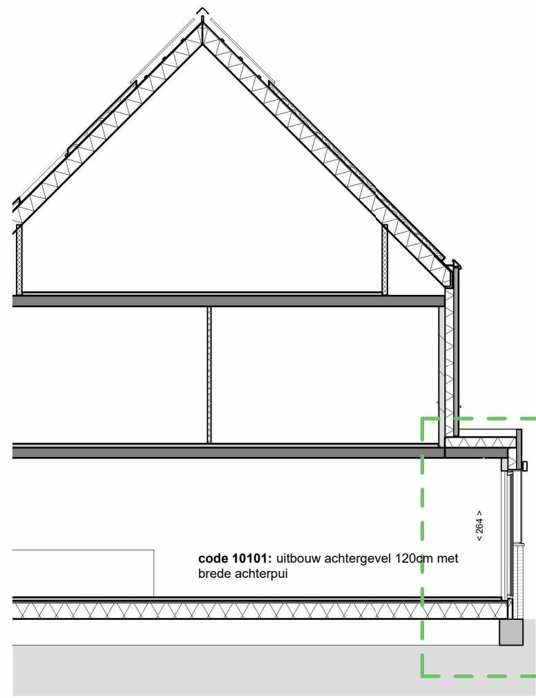
doorsnede
