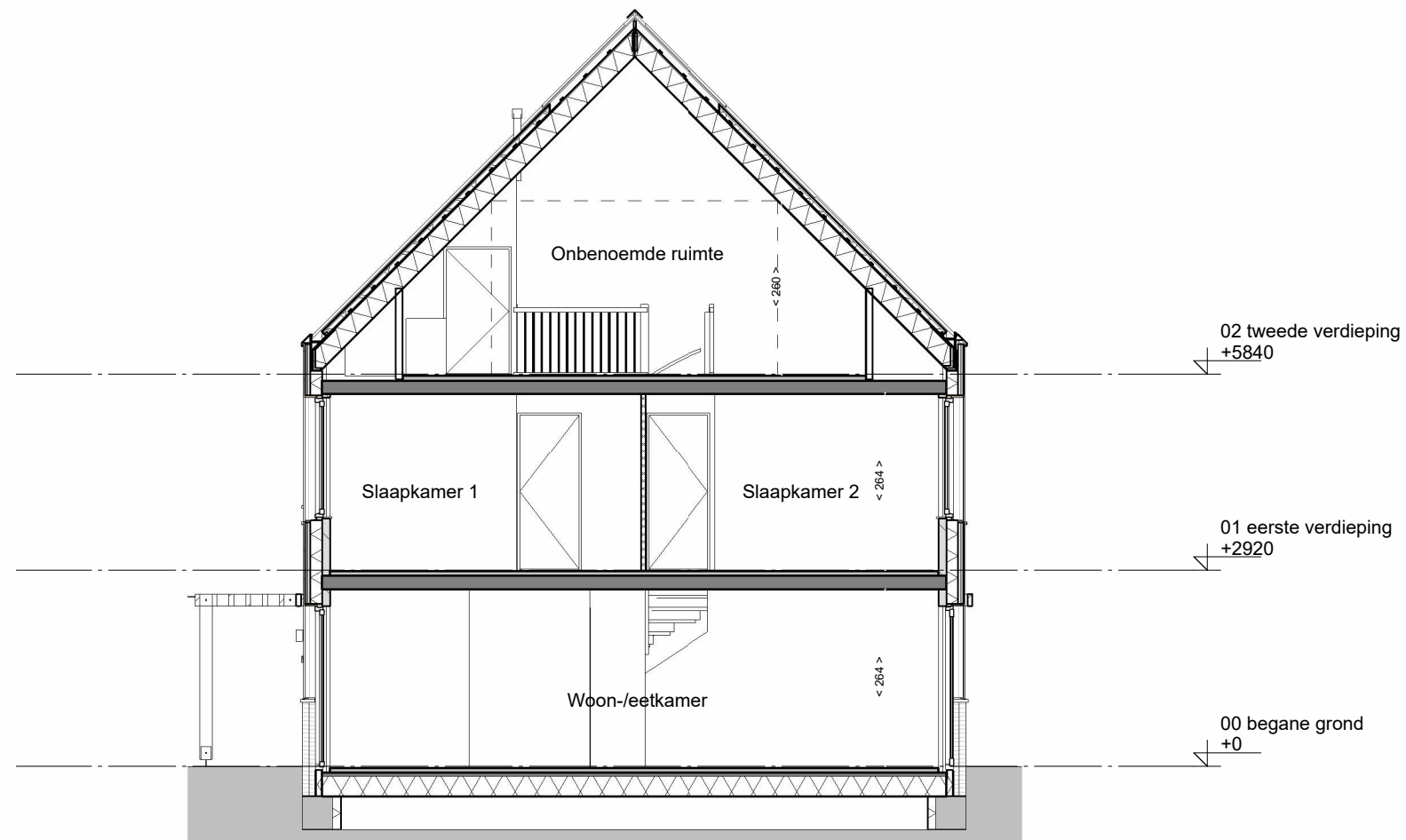
doorsnede
