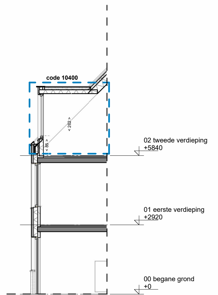
doorsnede
