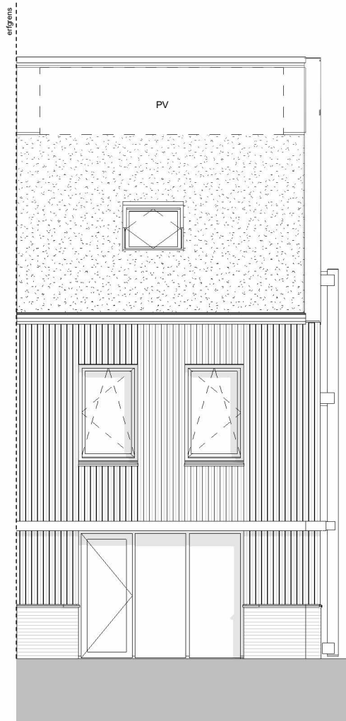
achtergevel
