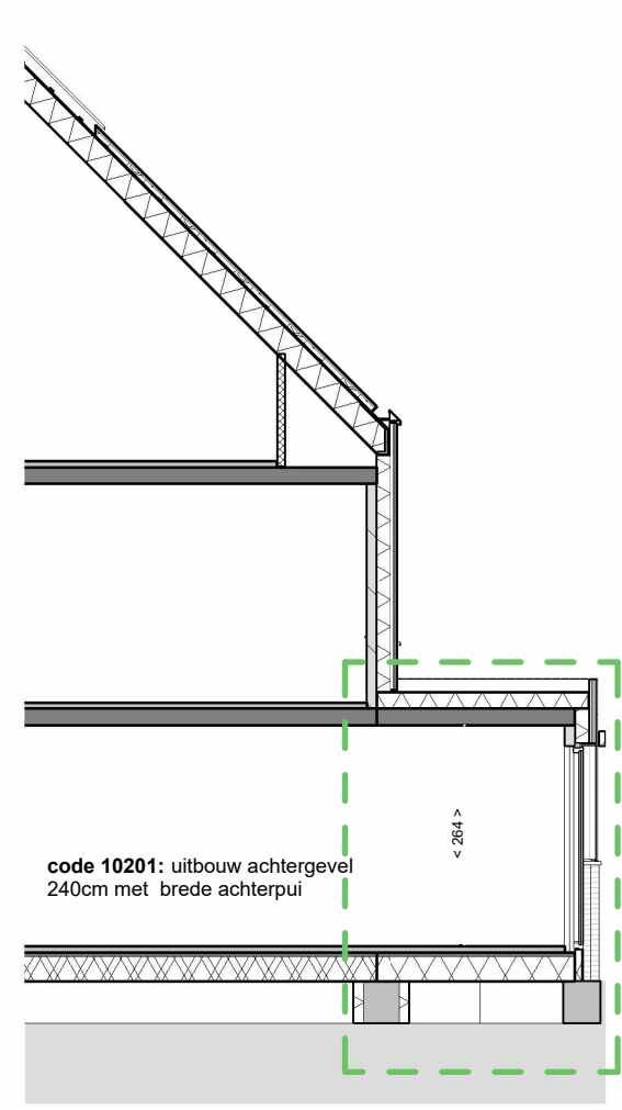
doorsnede
