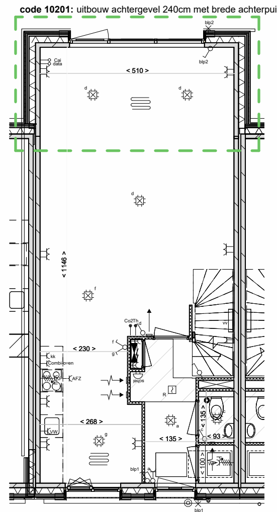
begane grond
